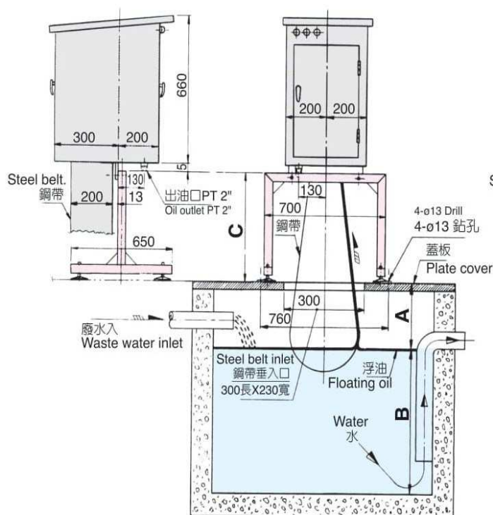
JF-50尺寸圖
